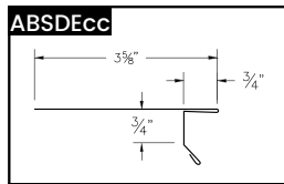
Drip Edge
